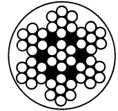
7 x 7 Wirelon
