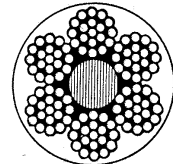
6 x 19 Wirelon
